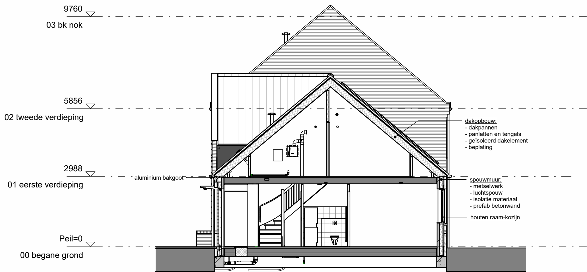
Doorsnede Bnr 109
