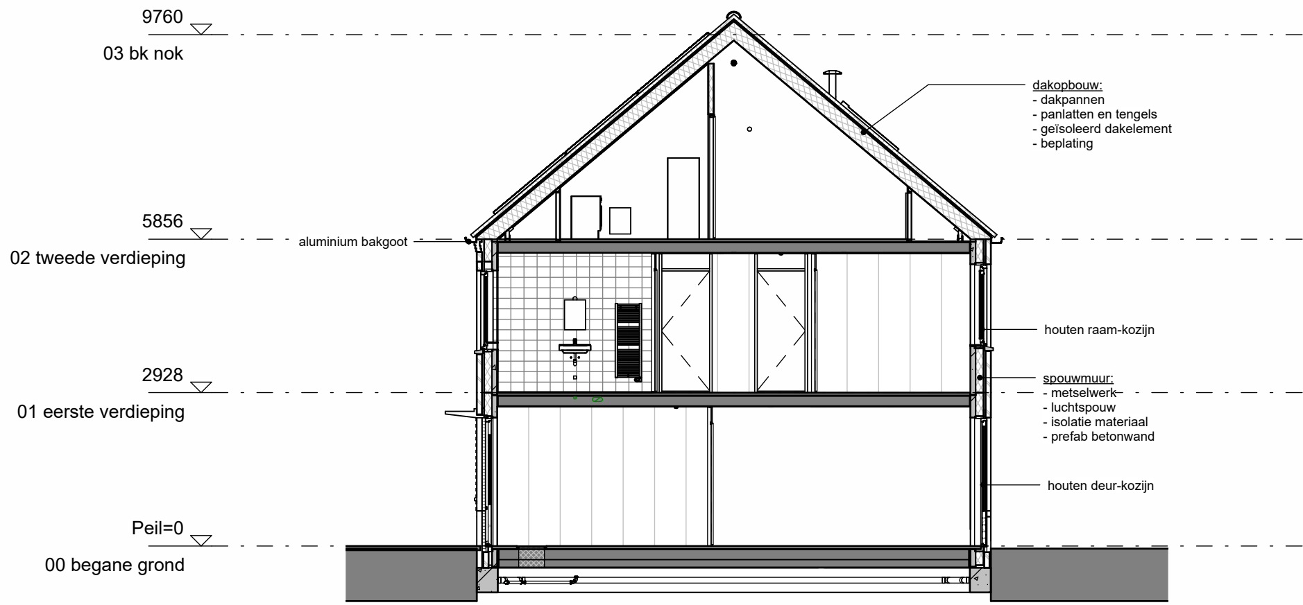
Doorsnede Bnr 108
