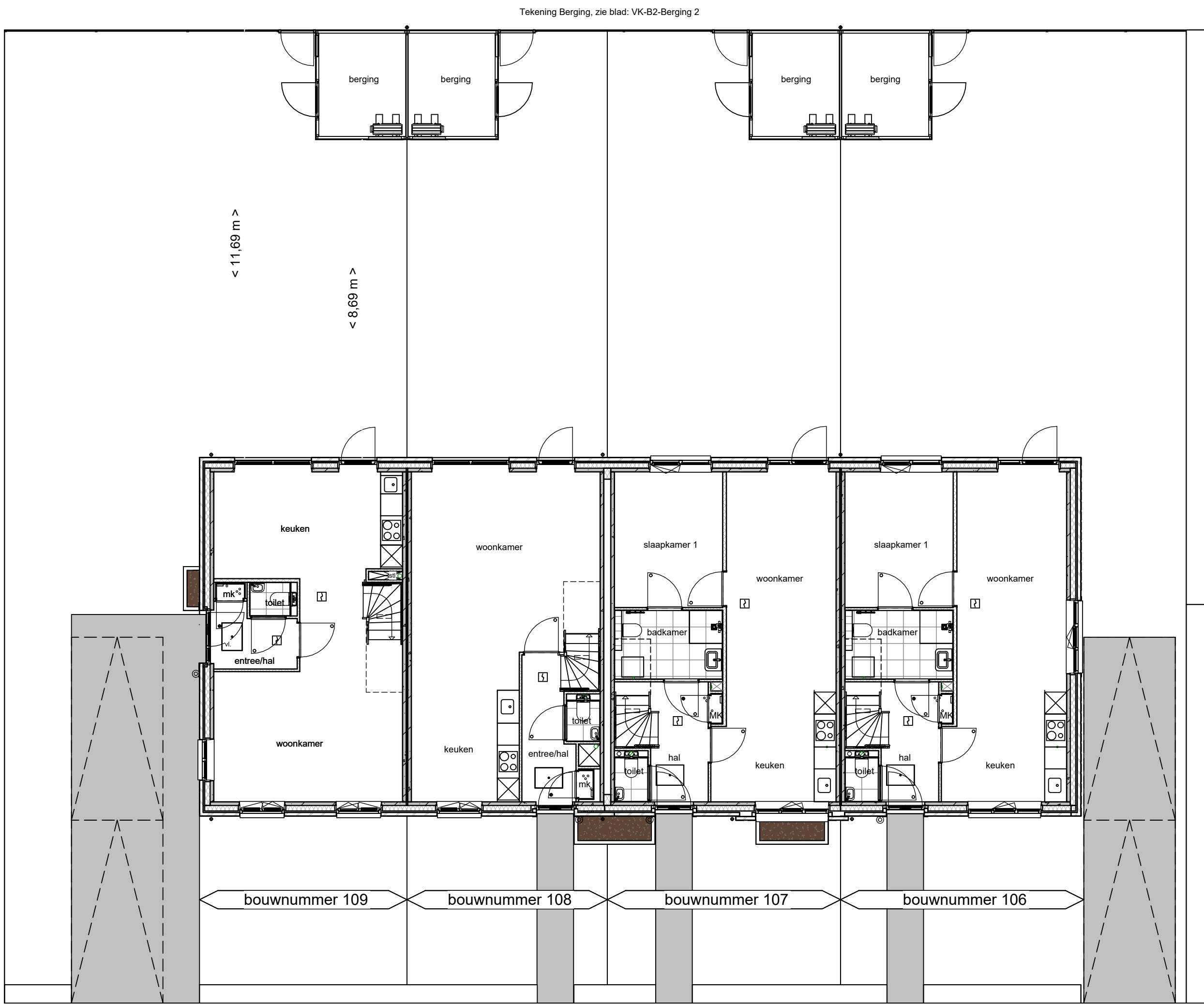
Begane grond
