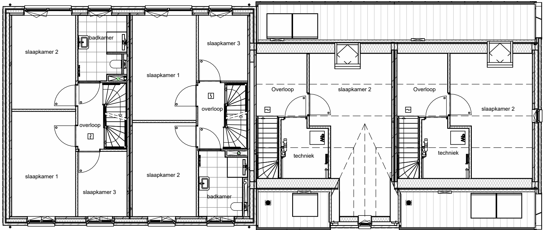
1e verdieping
