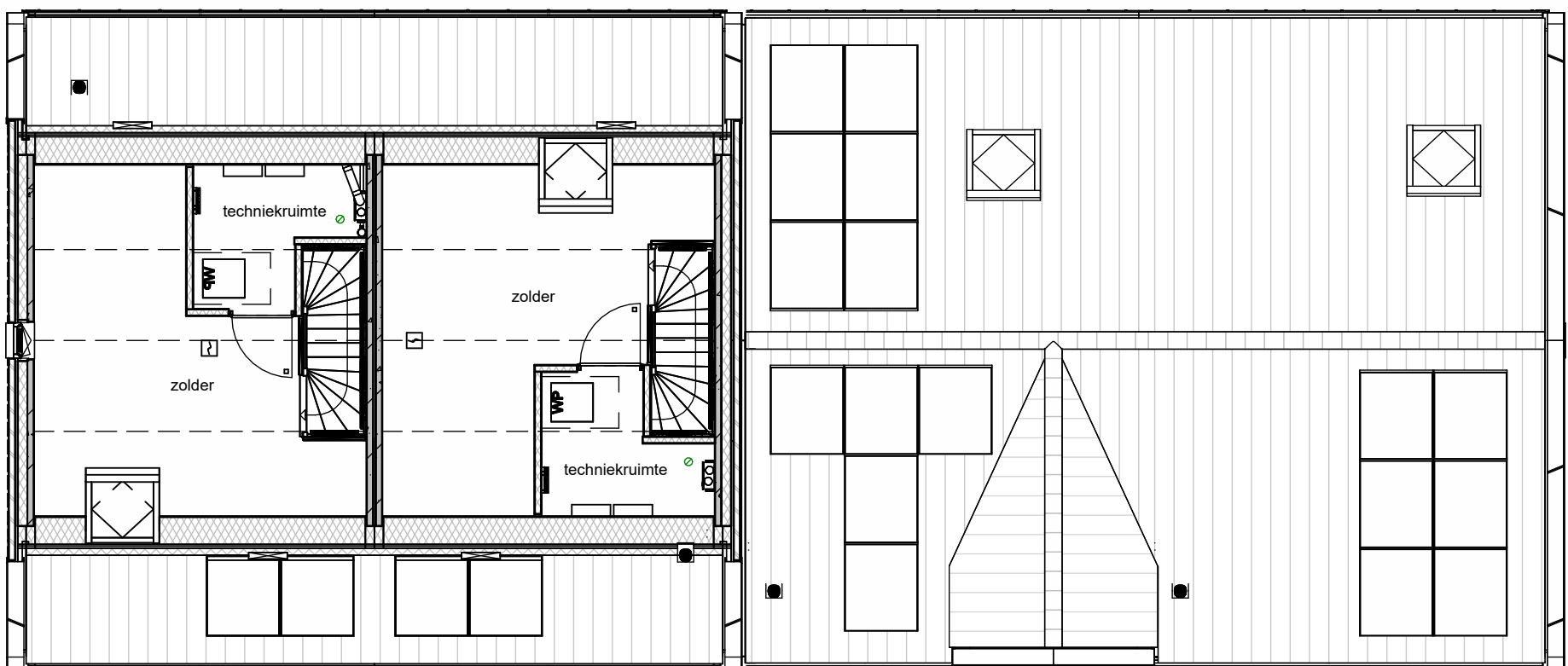
2e verdieping
