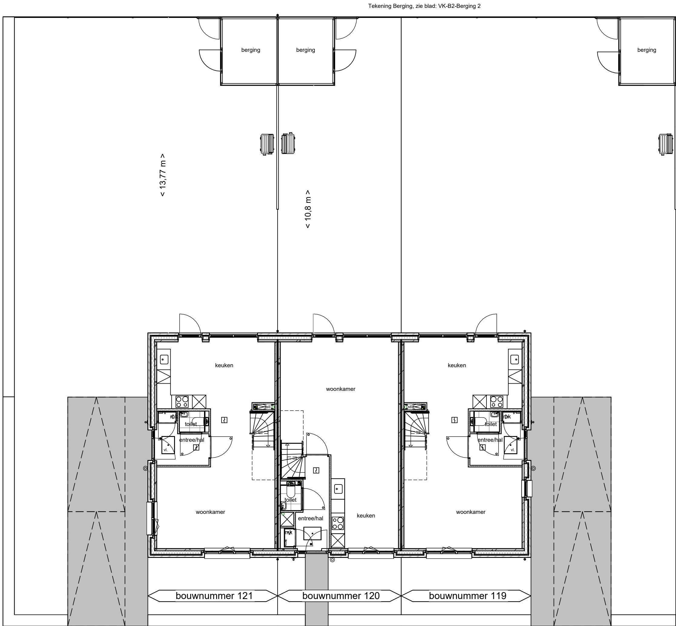
Begane grond
