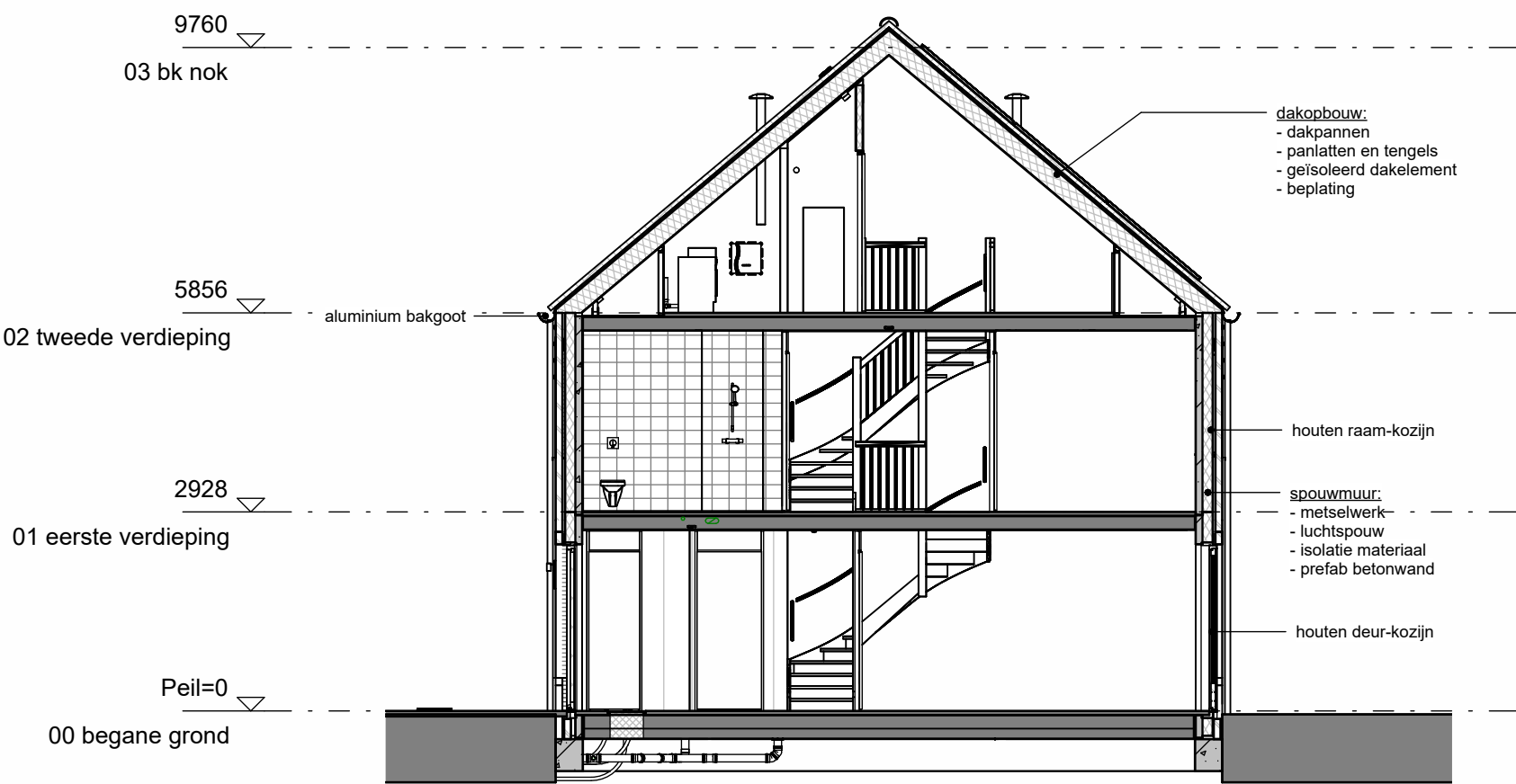
Doorsnede Bnr 120
