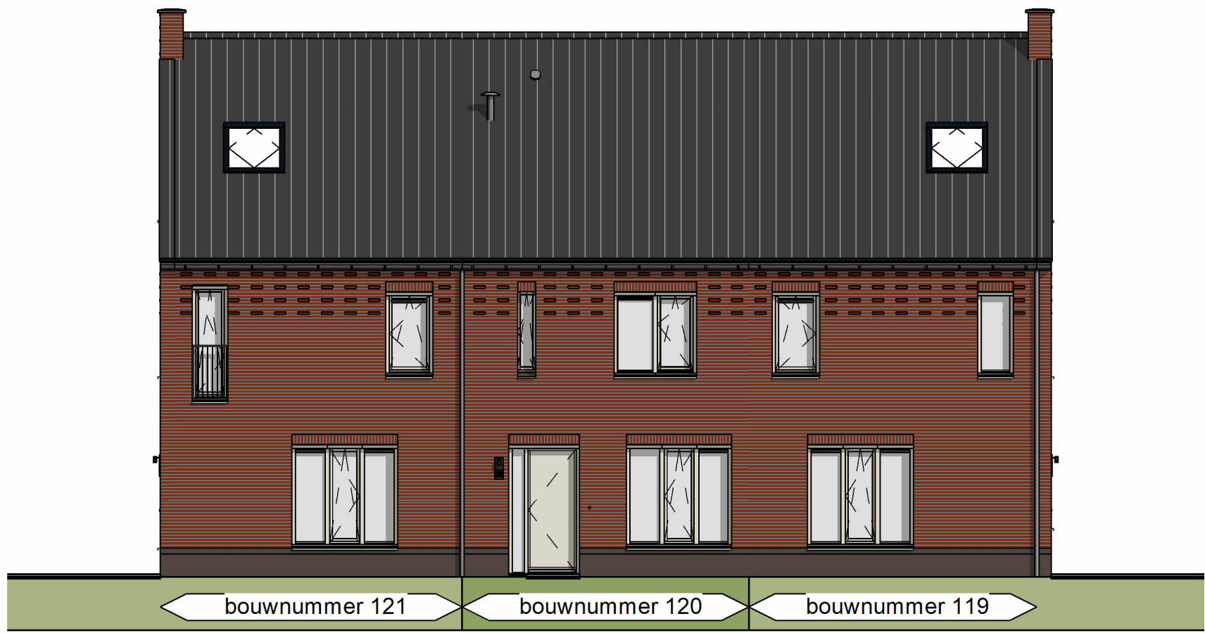
Voorgevel
