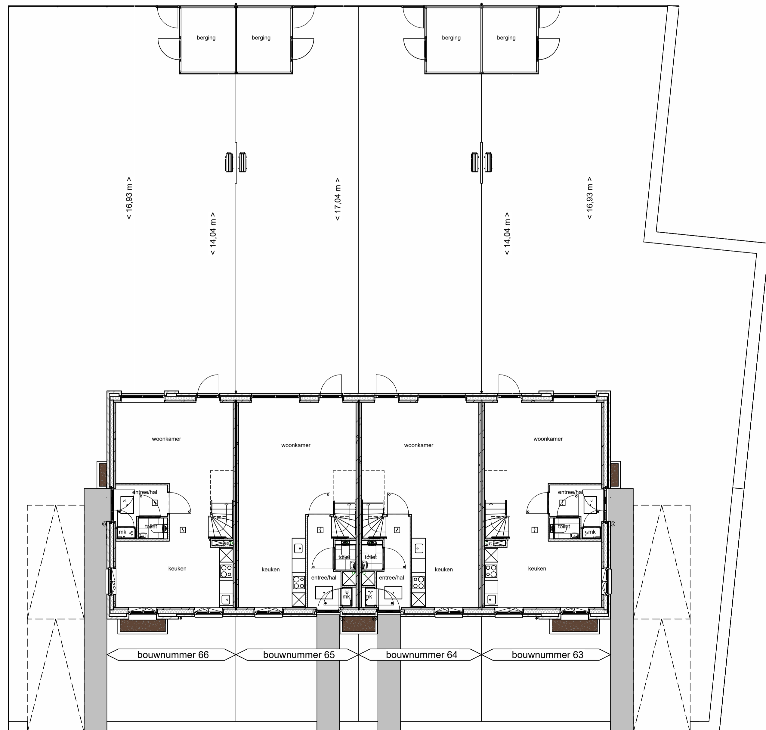
Begane grond
