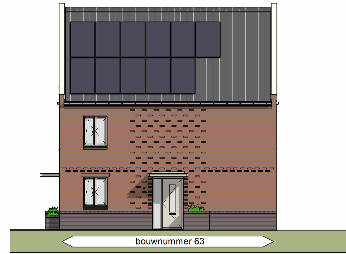
Rechter zijgevel
