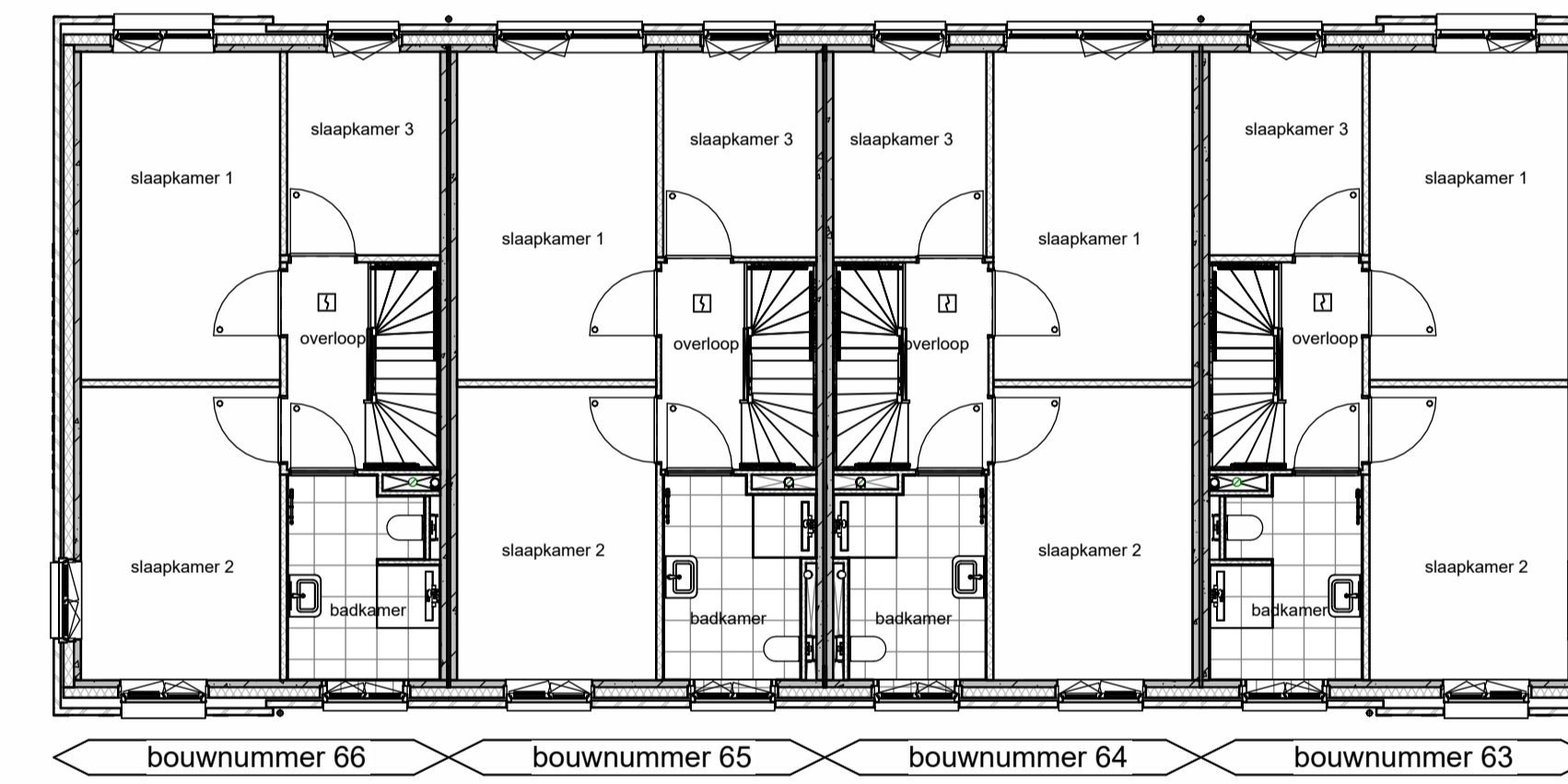
1e verdieping
