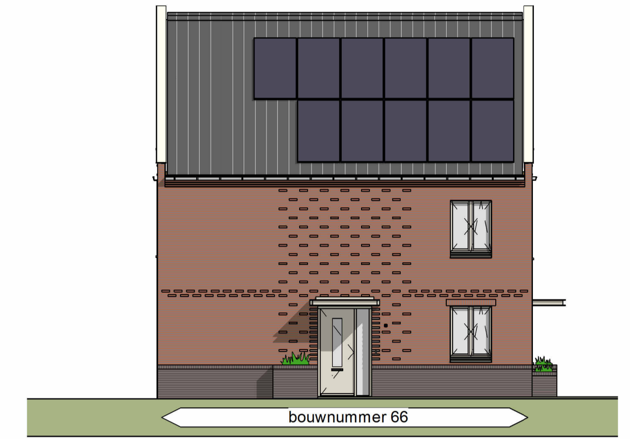
Linker zijgevel
