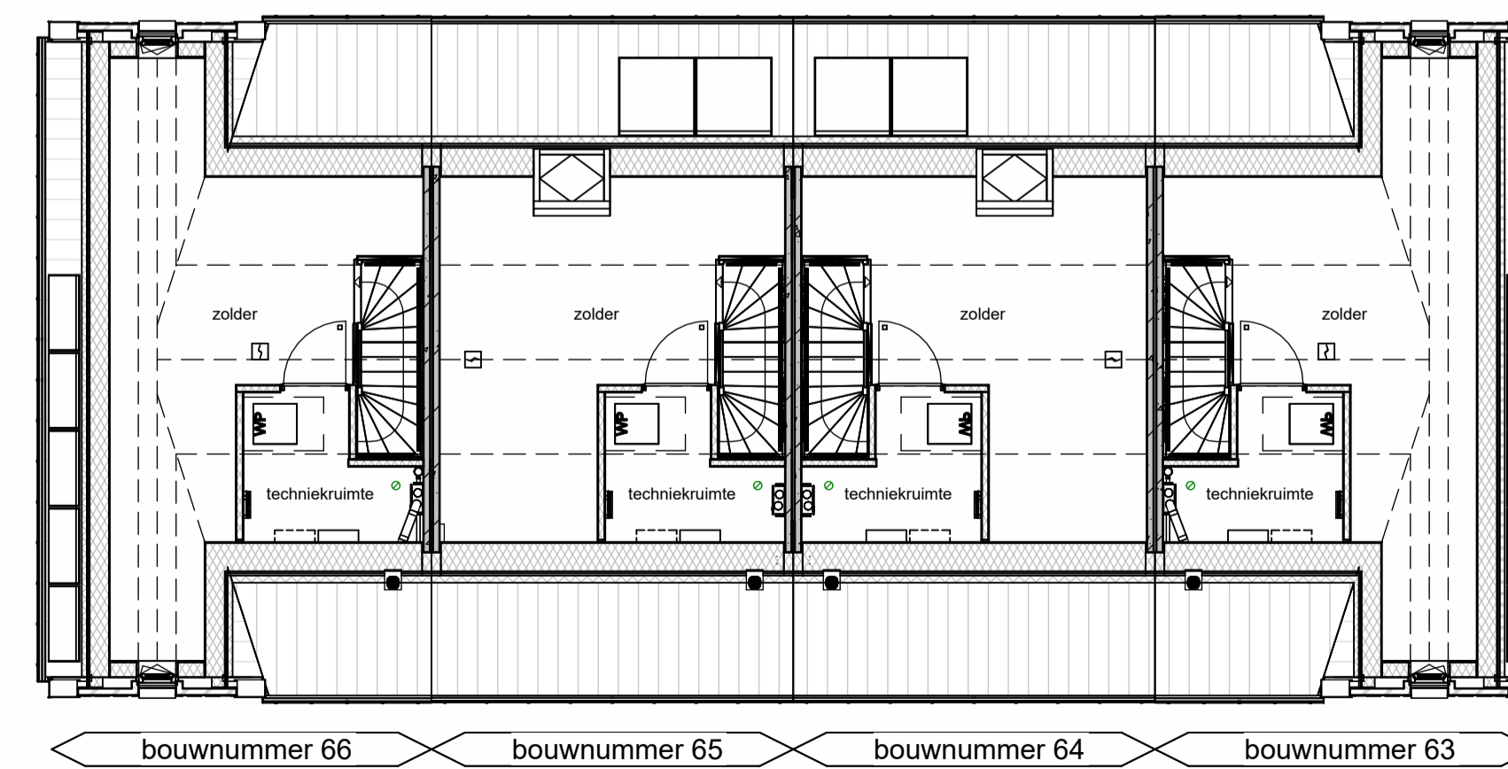
2e verdieping
