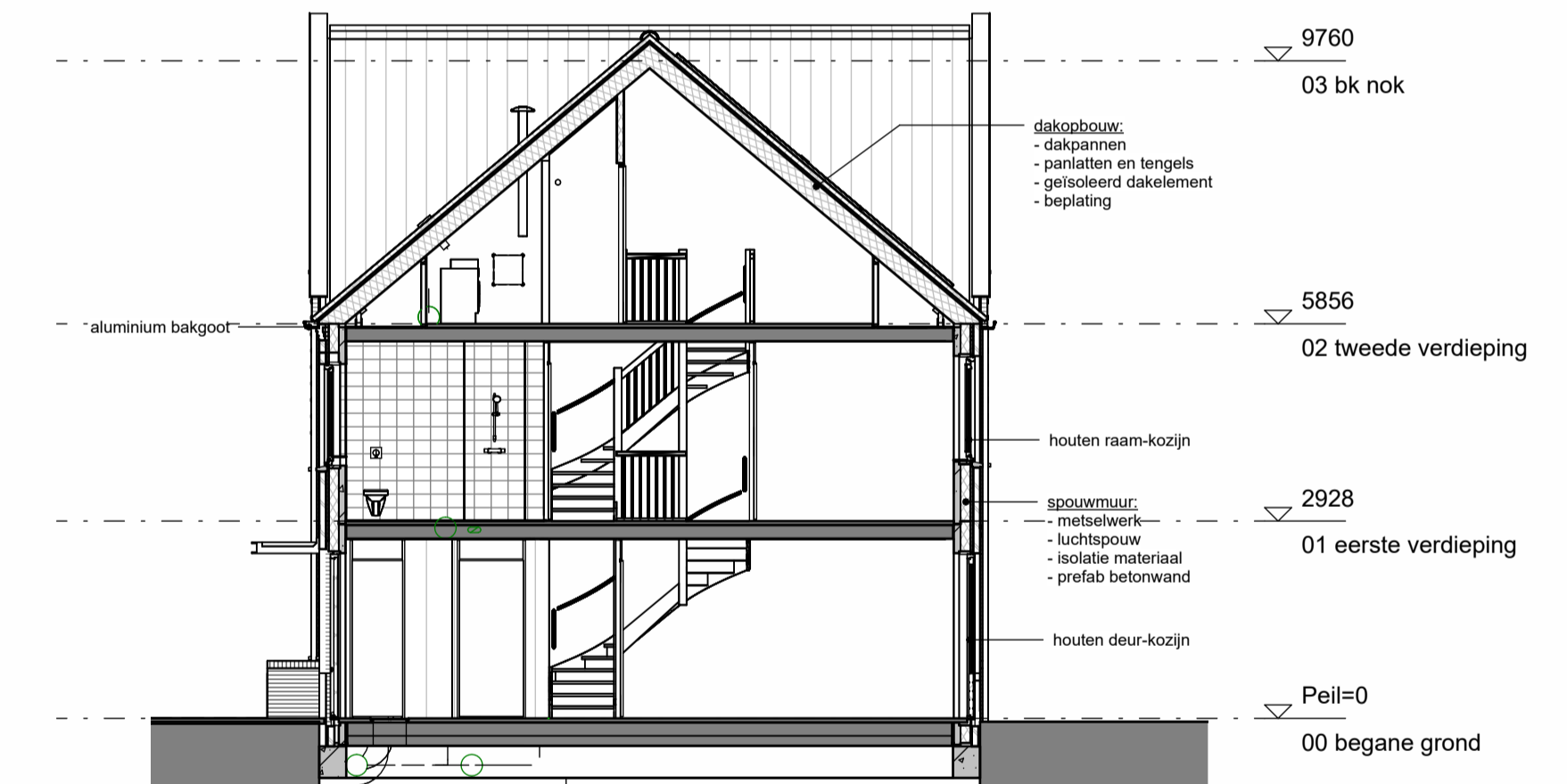
Doorsnede
