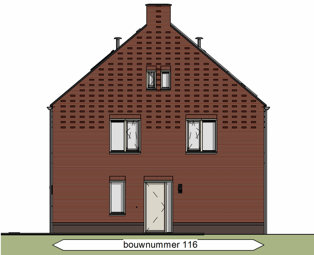
Rechter zijgevel
