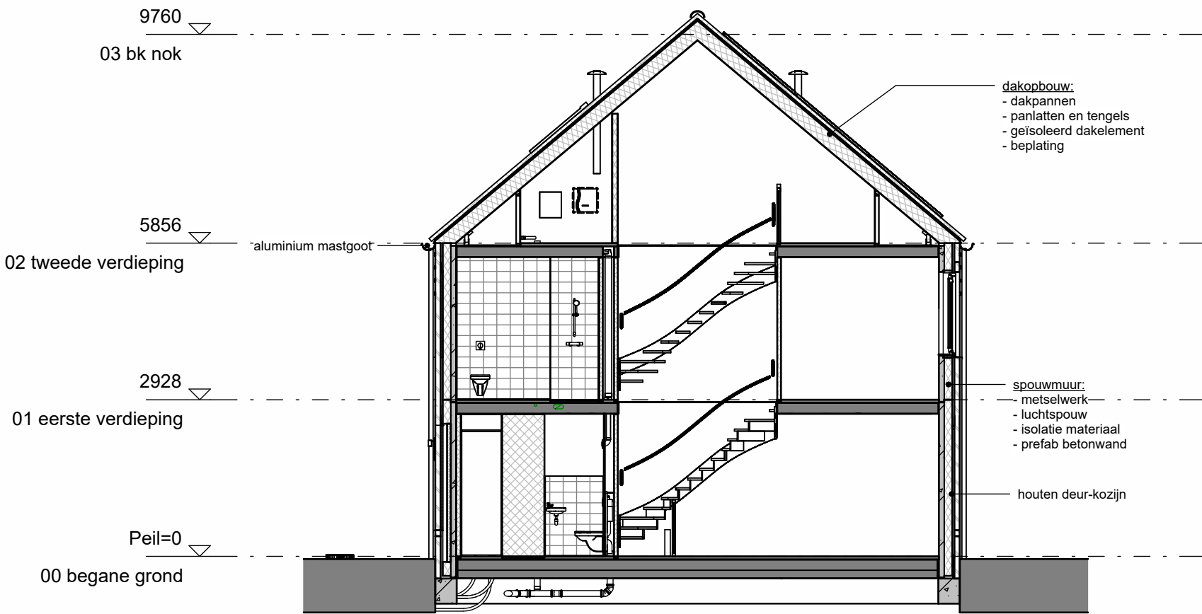
Doorsnede Bnr 117
