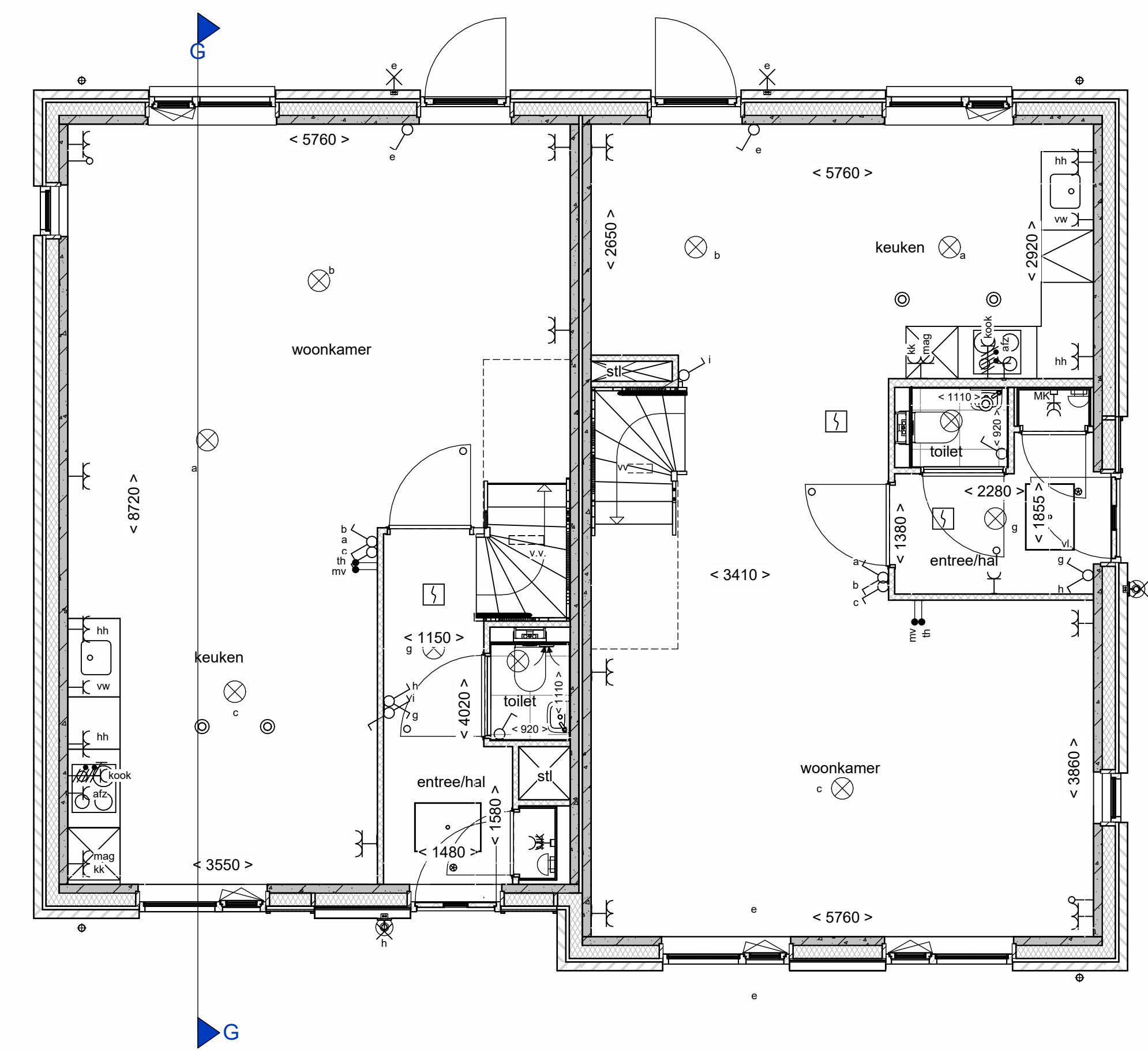
Begane grond
