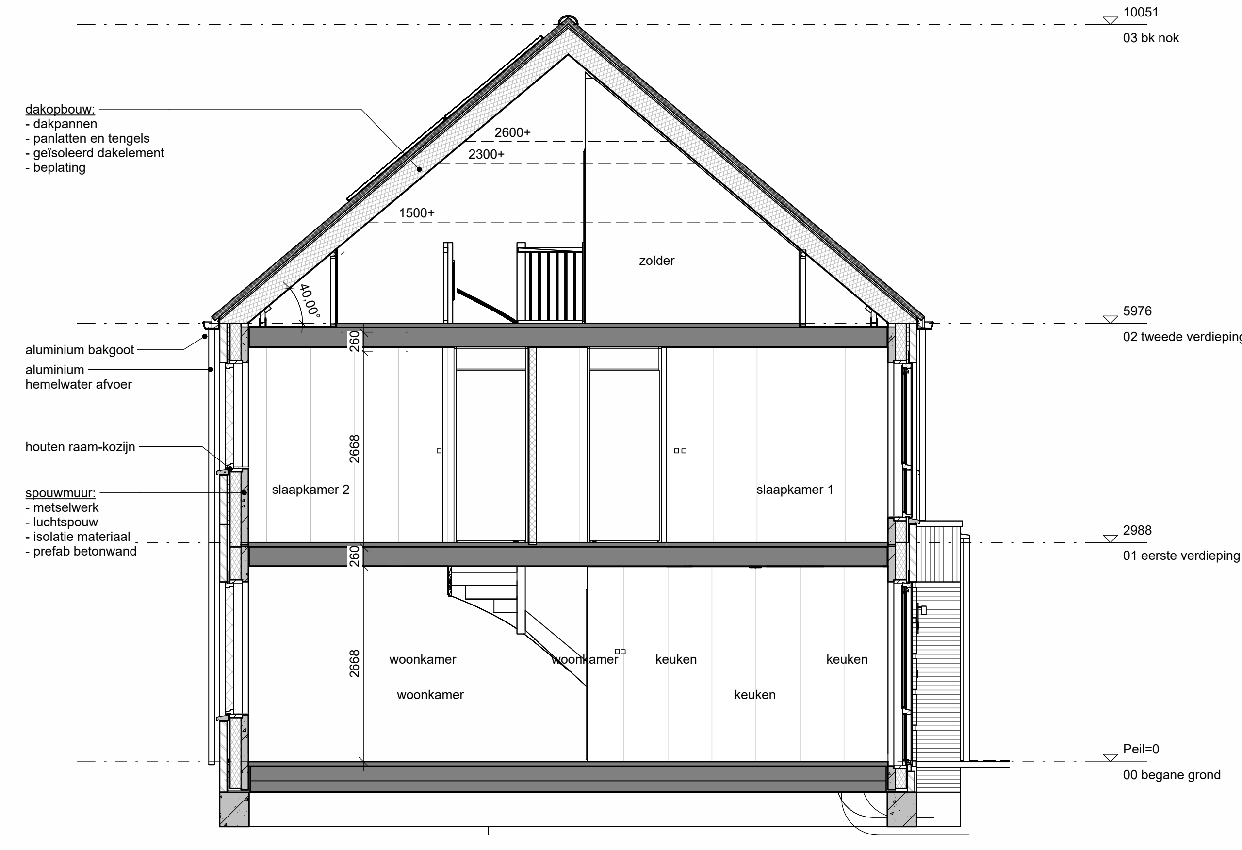
doorsnede G
