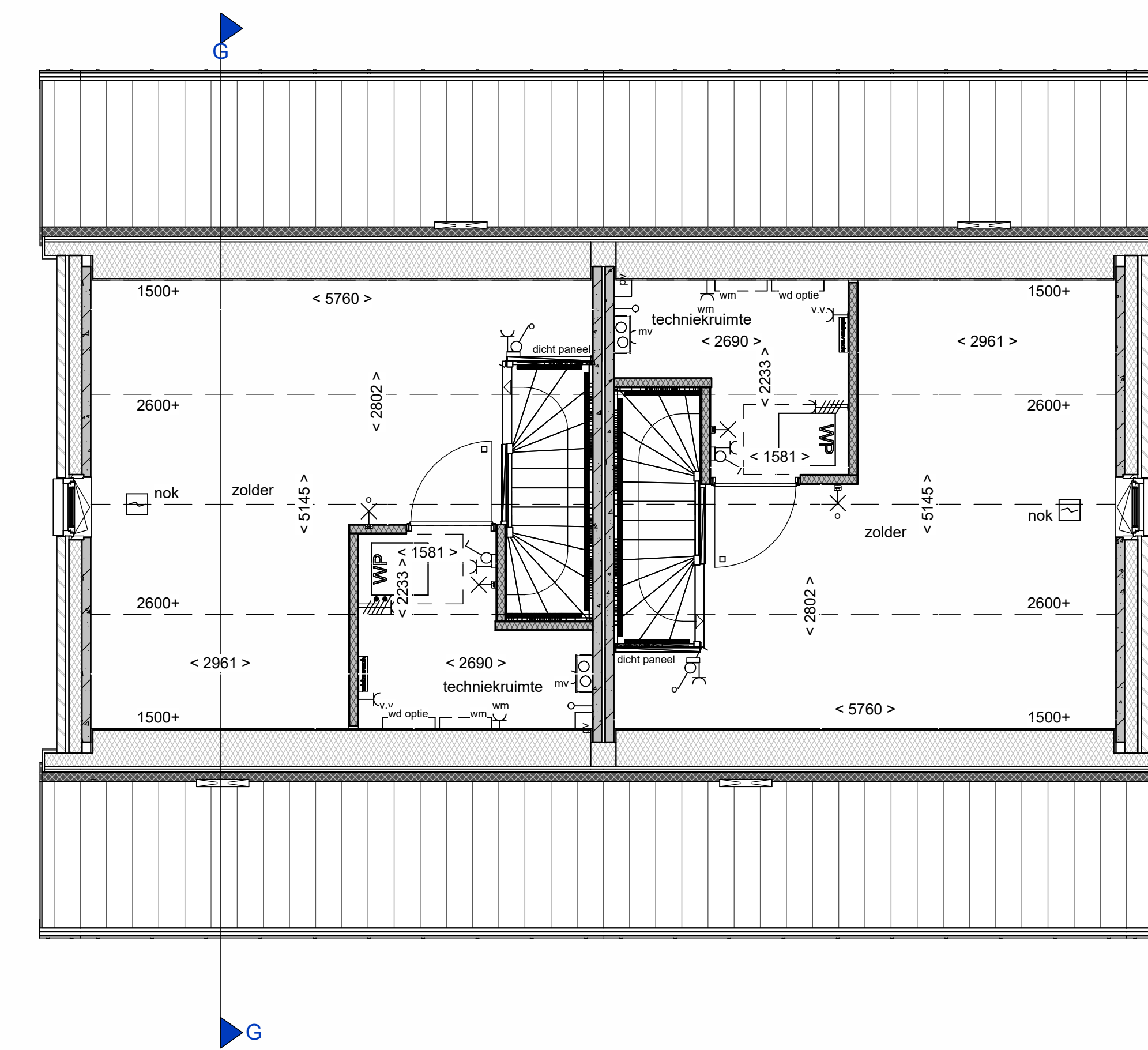
2e verdieping
