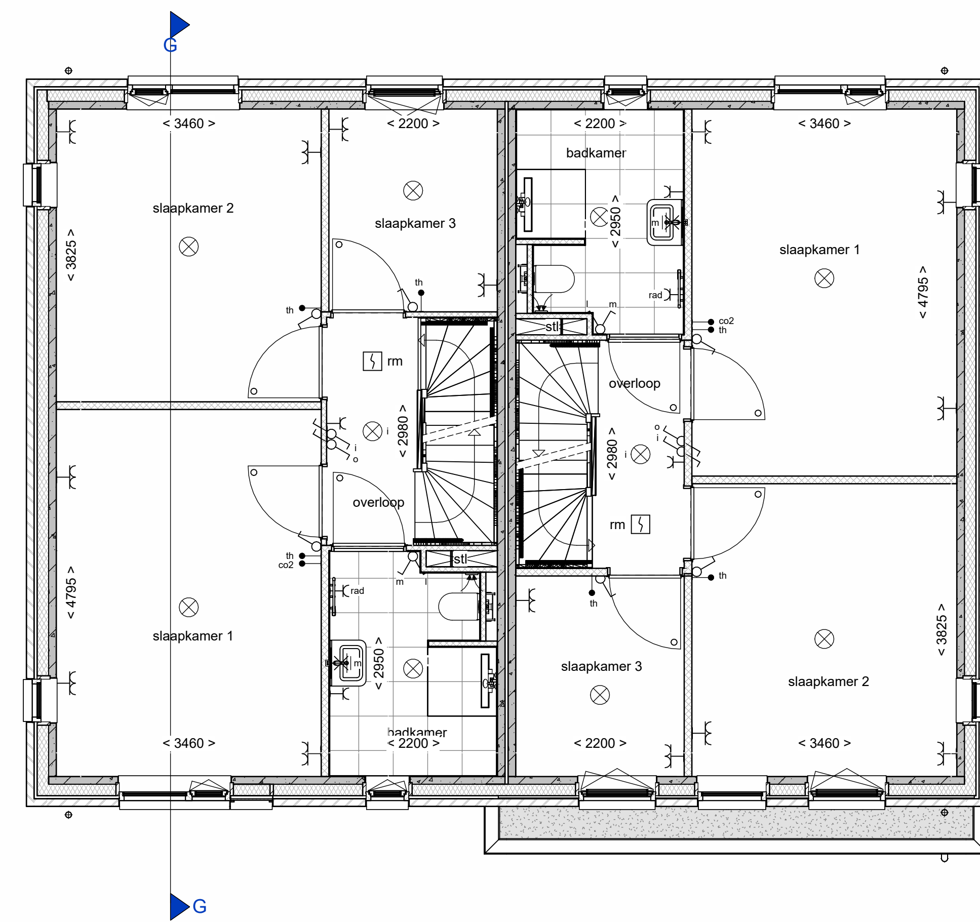
1e verdieping
