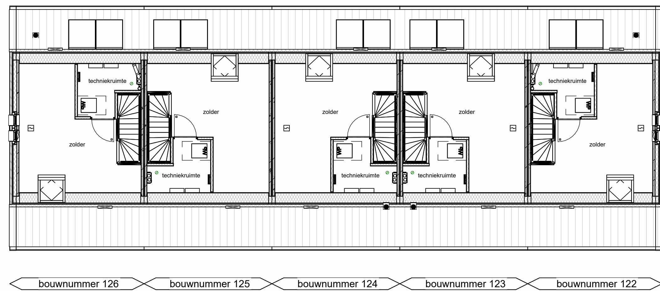
2e verdieping
