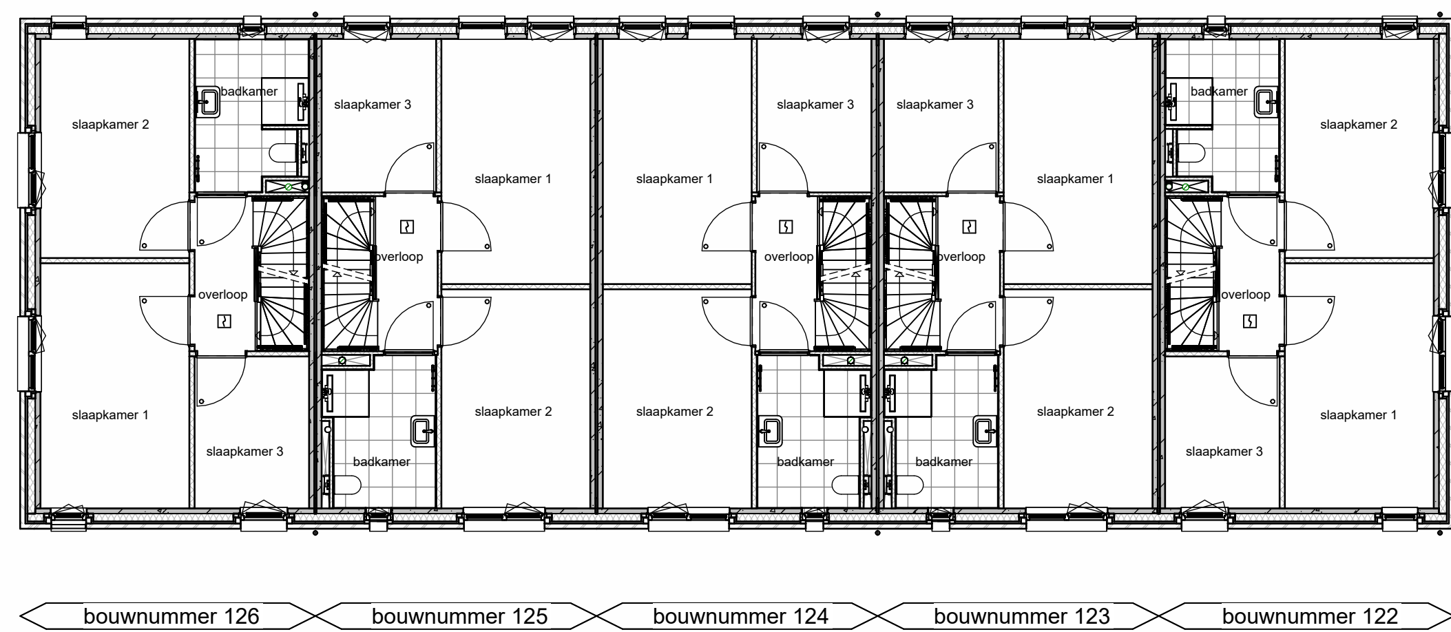
1e verdieping
