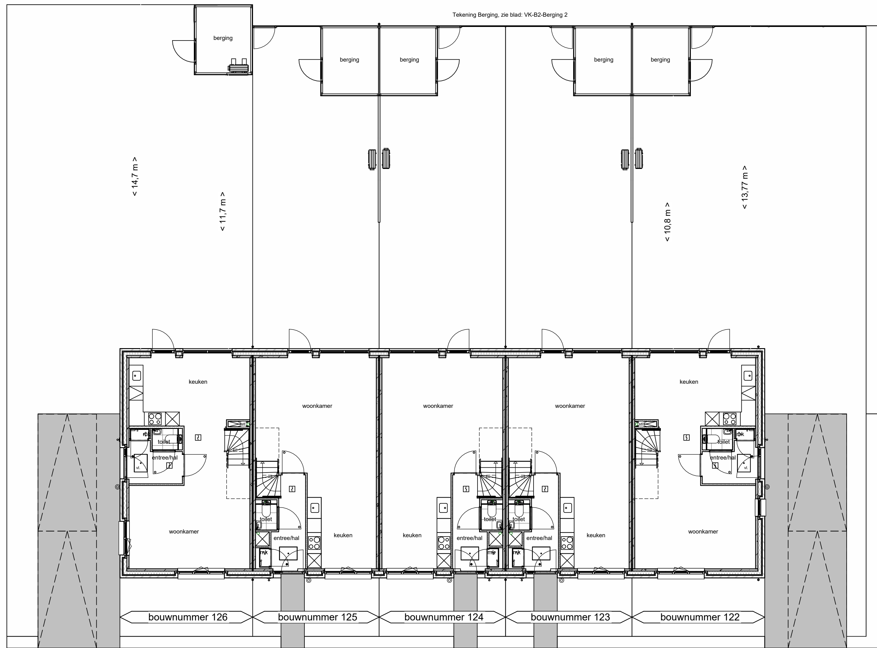
Begane grond
