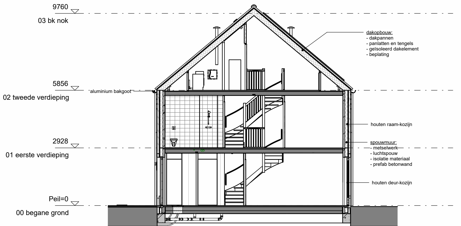
Doorsnede Bnr 125
