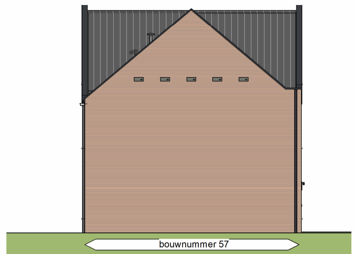
Linker zijgevel
