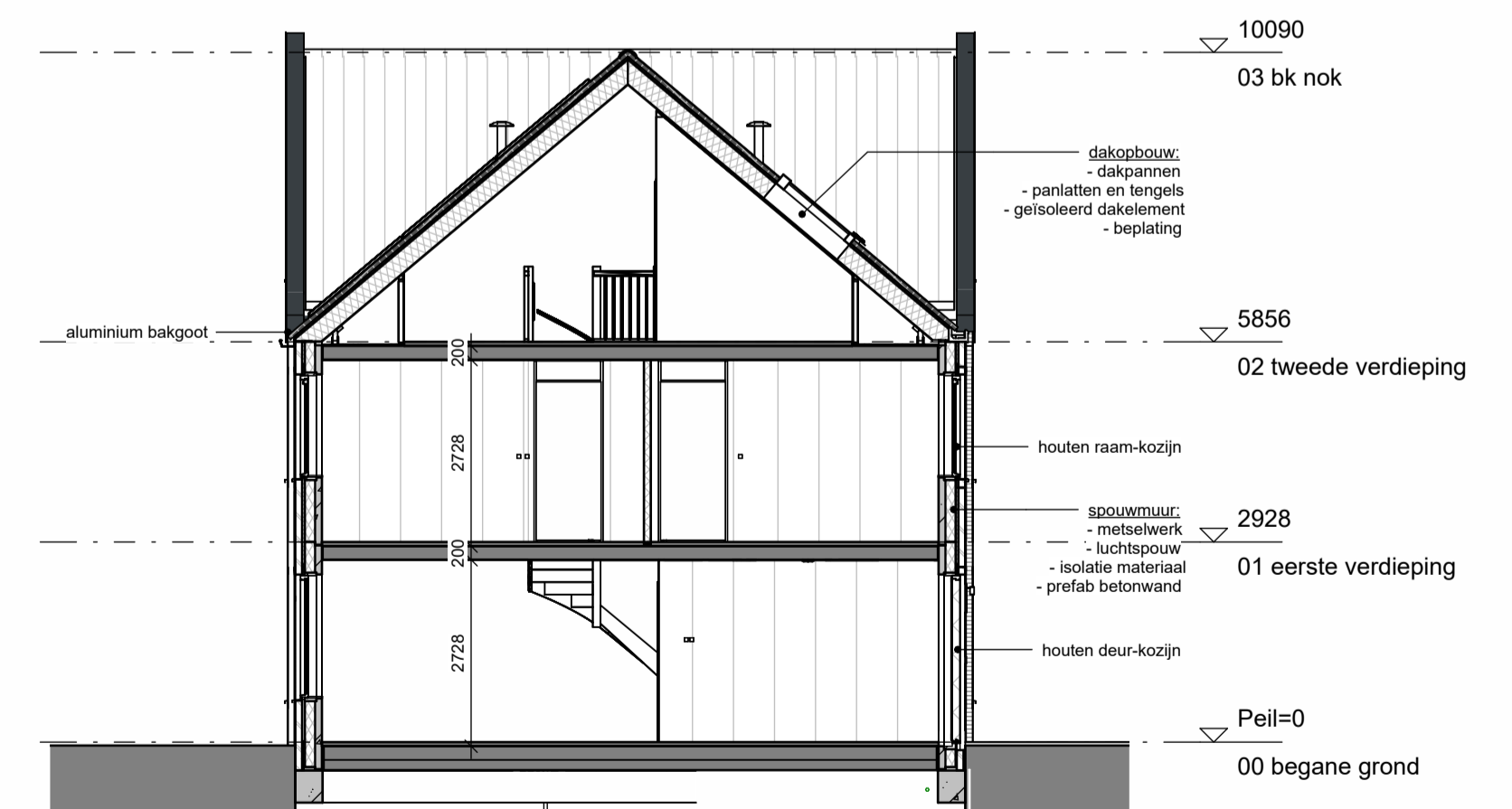
Doorsnede Bnr 55.57
