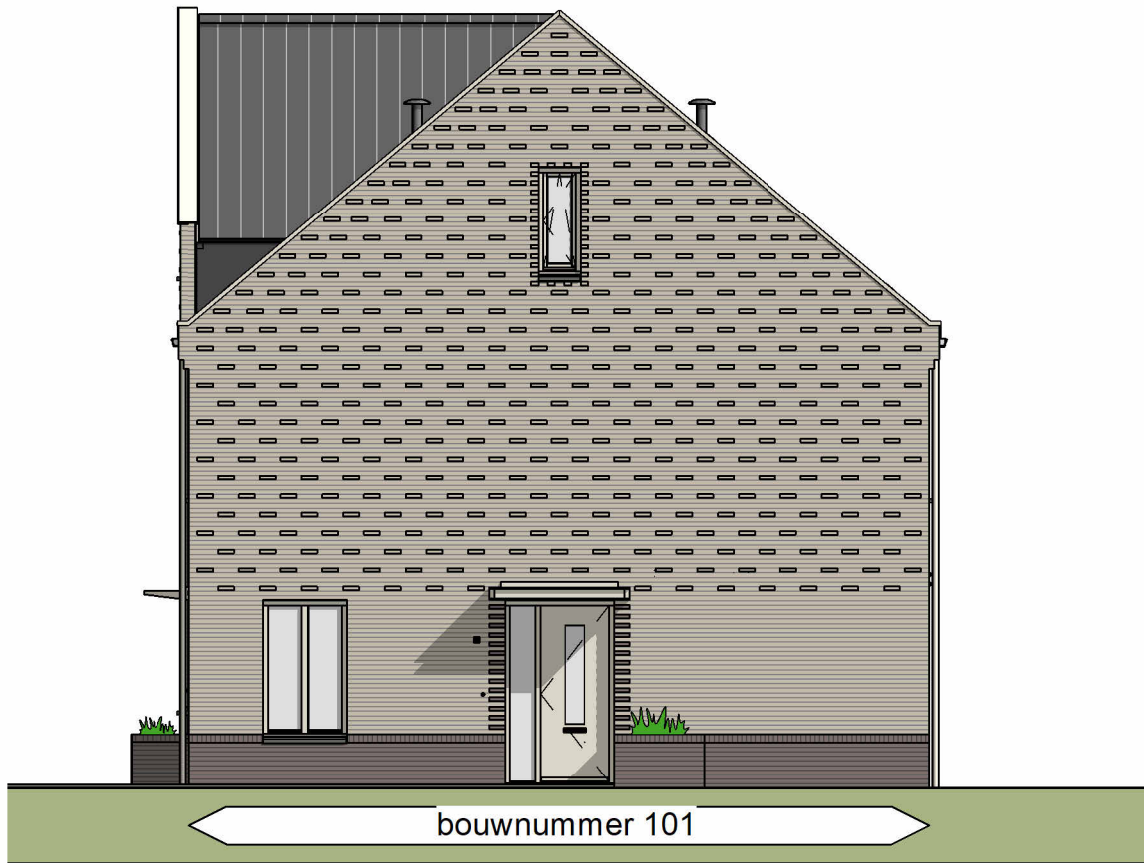
Rechter zijgevel
