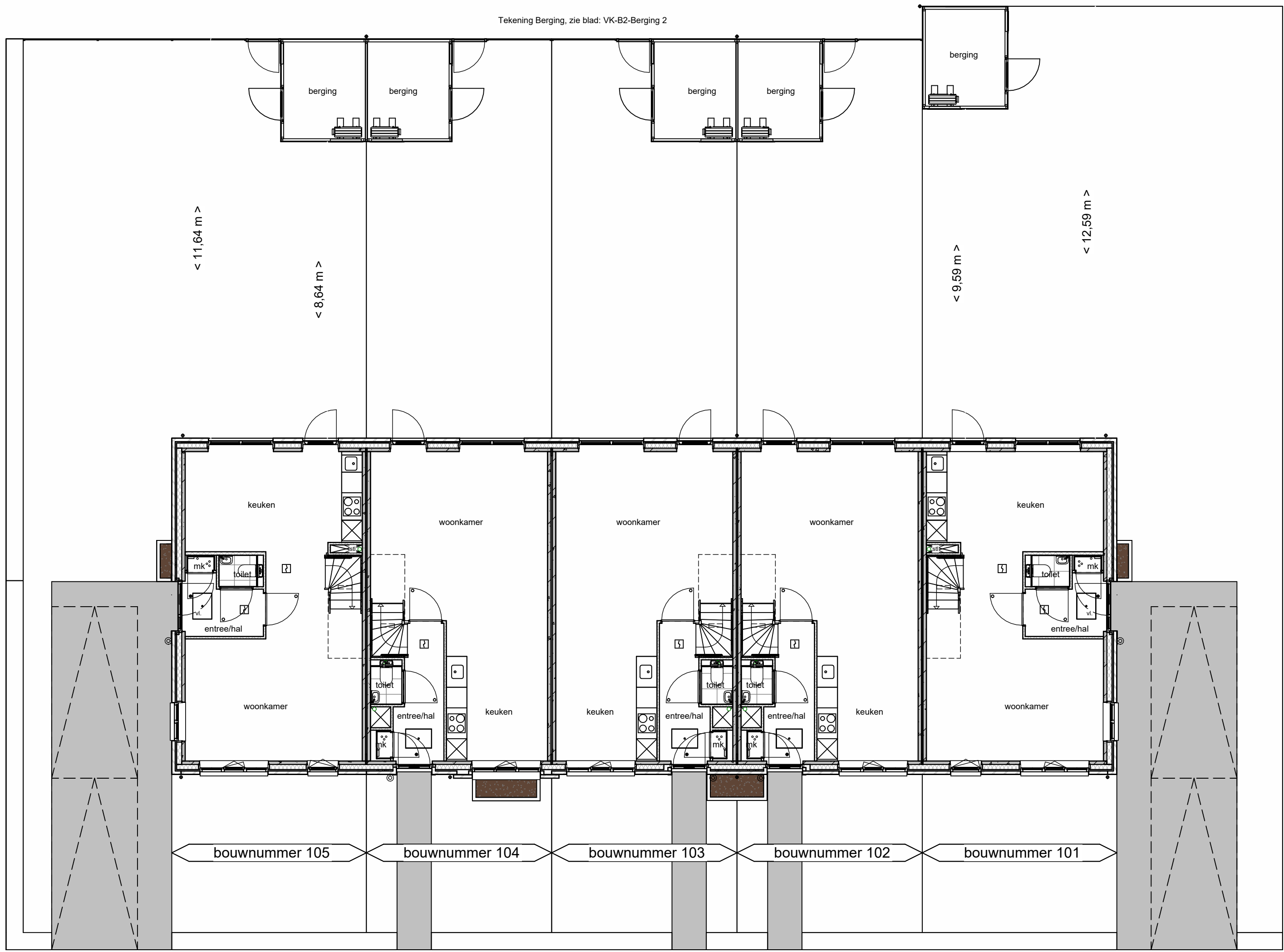
Begane grond
