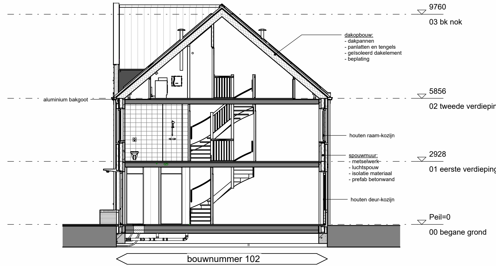
Doorsnede
