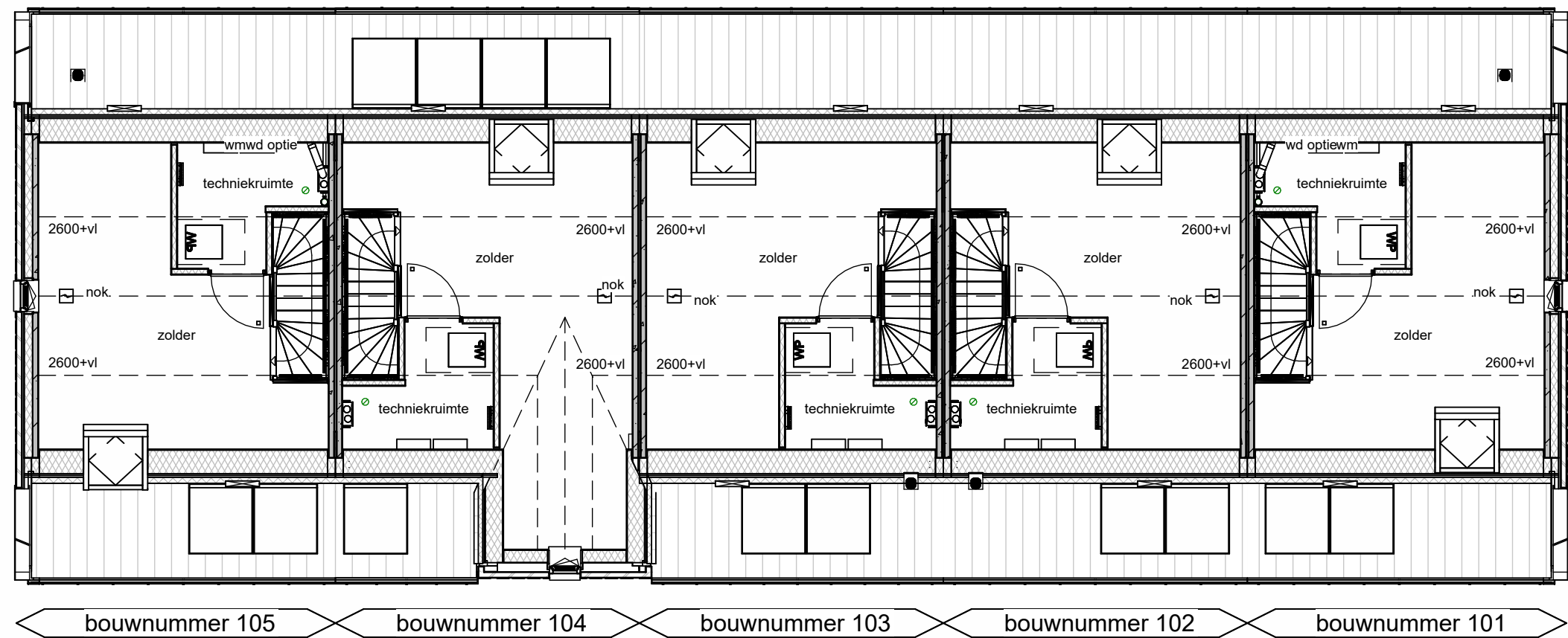
2e verdieping
