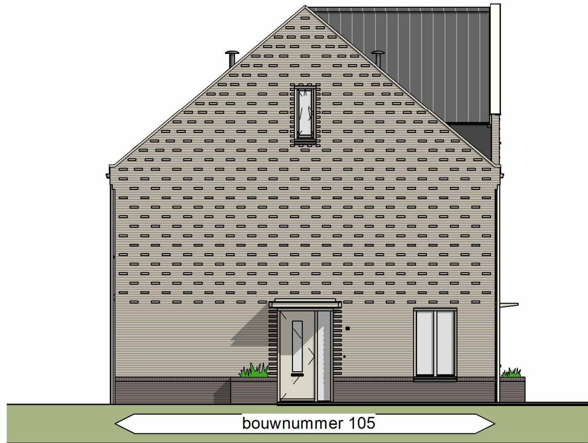
Linker zijgevel
