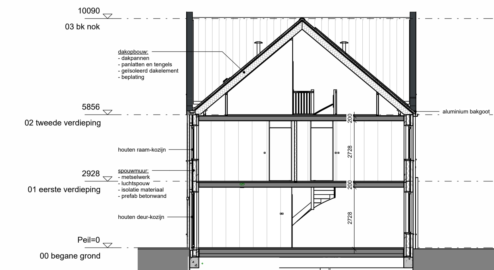
Doorsnede Bnr 58.62
