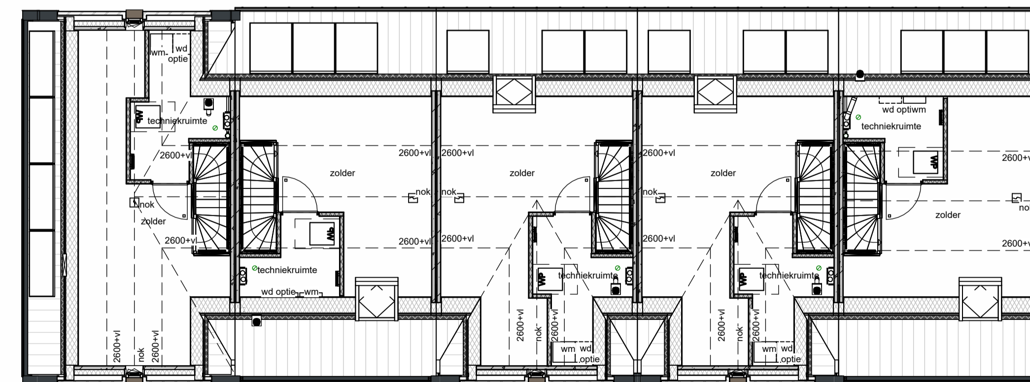
2e verdieping
