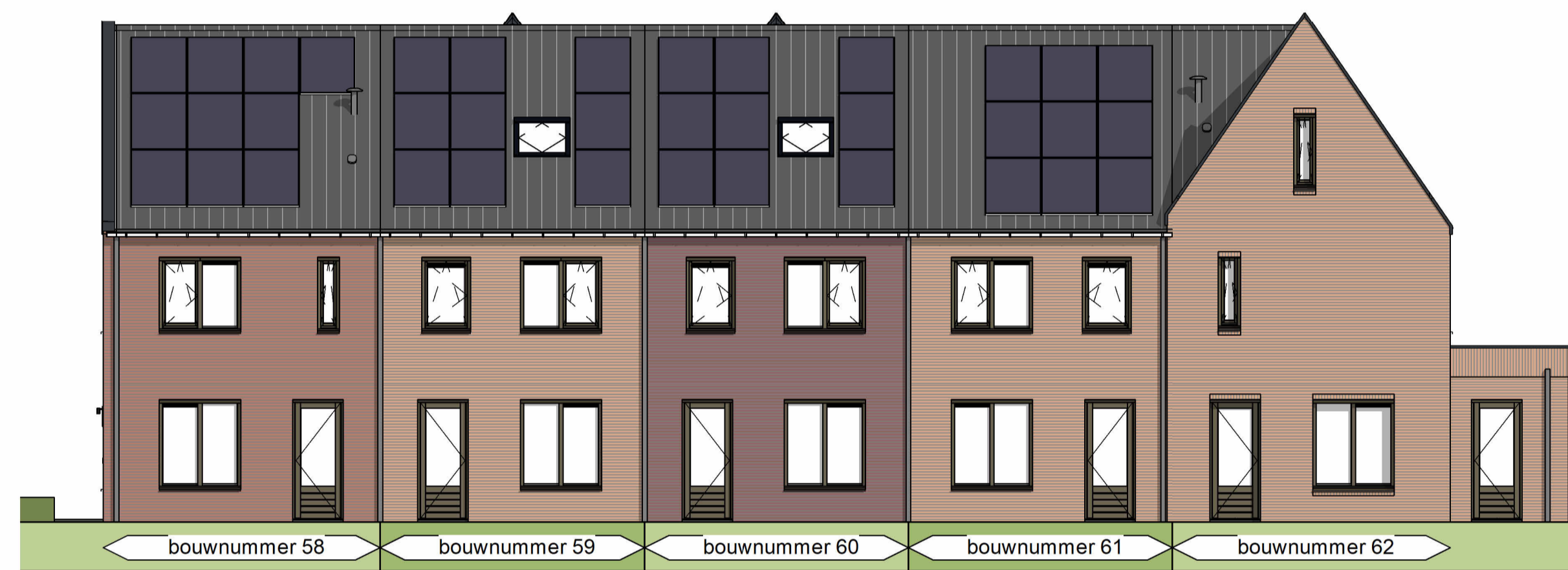
Achtergevel
