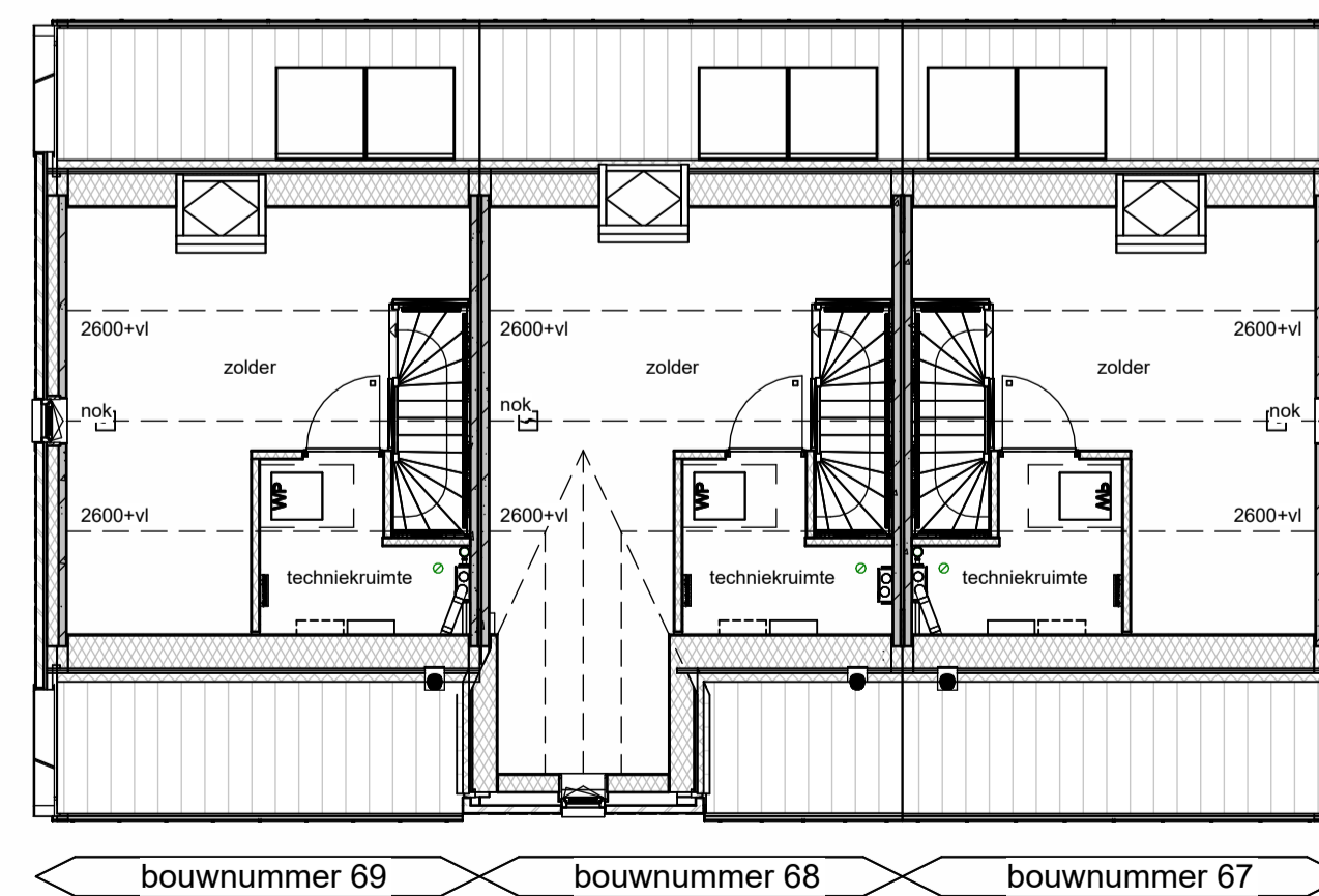
2e verdieping
