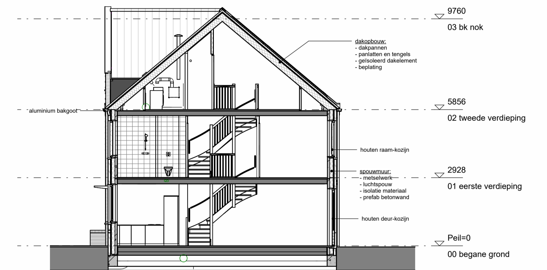
Doorsnede
