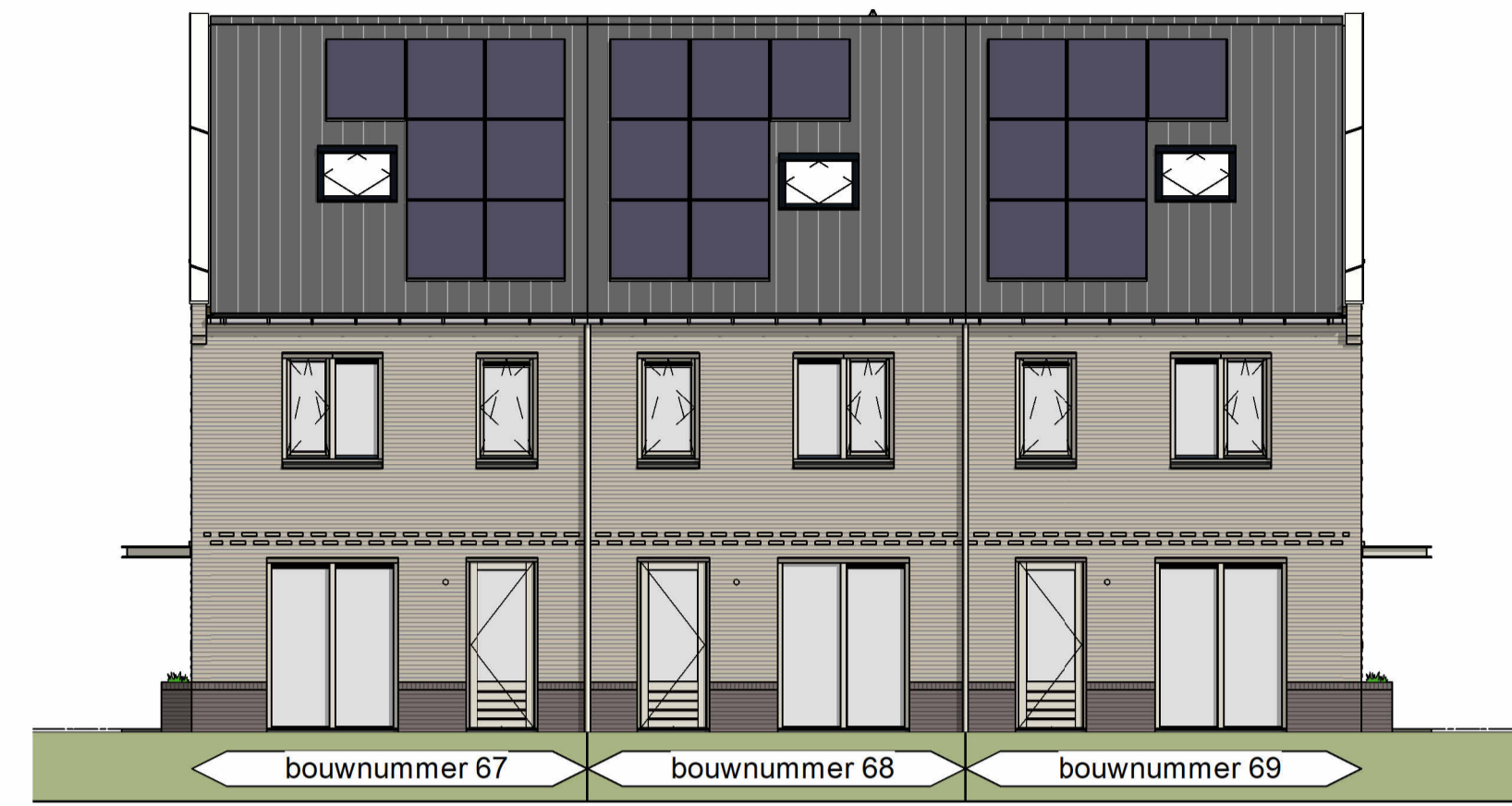
Achtergevel
