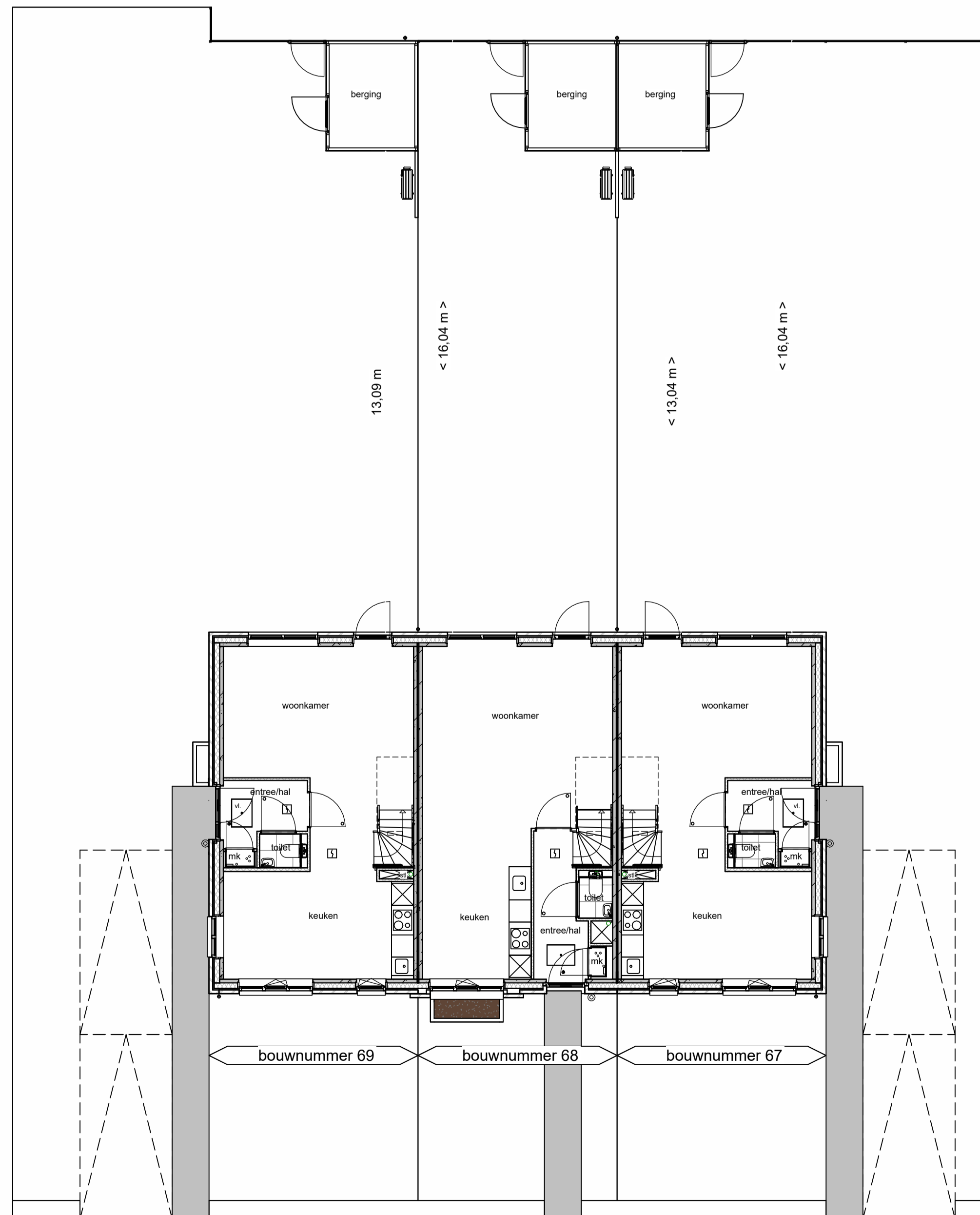
Begane grond
